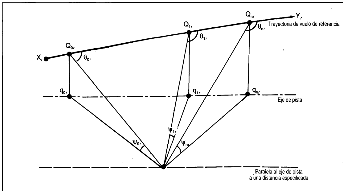
Figura 2-15 b). Trayectoria de vuelo de referencia
