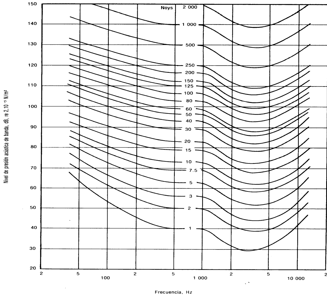
Figura 5-1. Curvas de ruidosidad percibida
